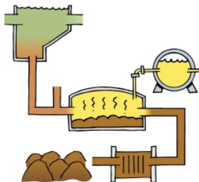
Slam fra 1. rensetrin til rådnetank og kompostering Sludge from primary treatment to the digester and then compost production
