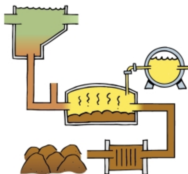
Slam fra 1. rensesettrin til rådnetank og kompostering Sludge from primary treatment to the digester and then compost production
