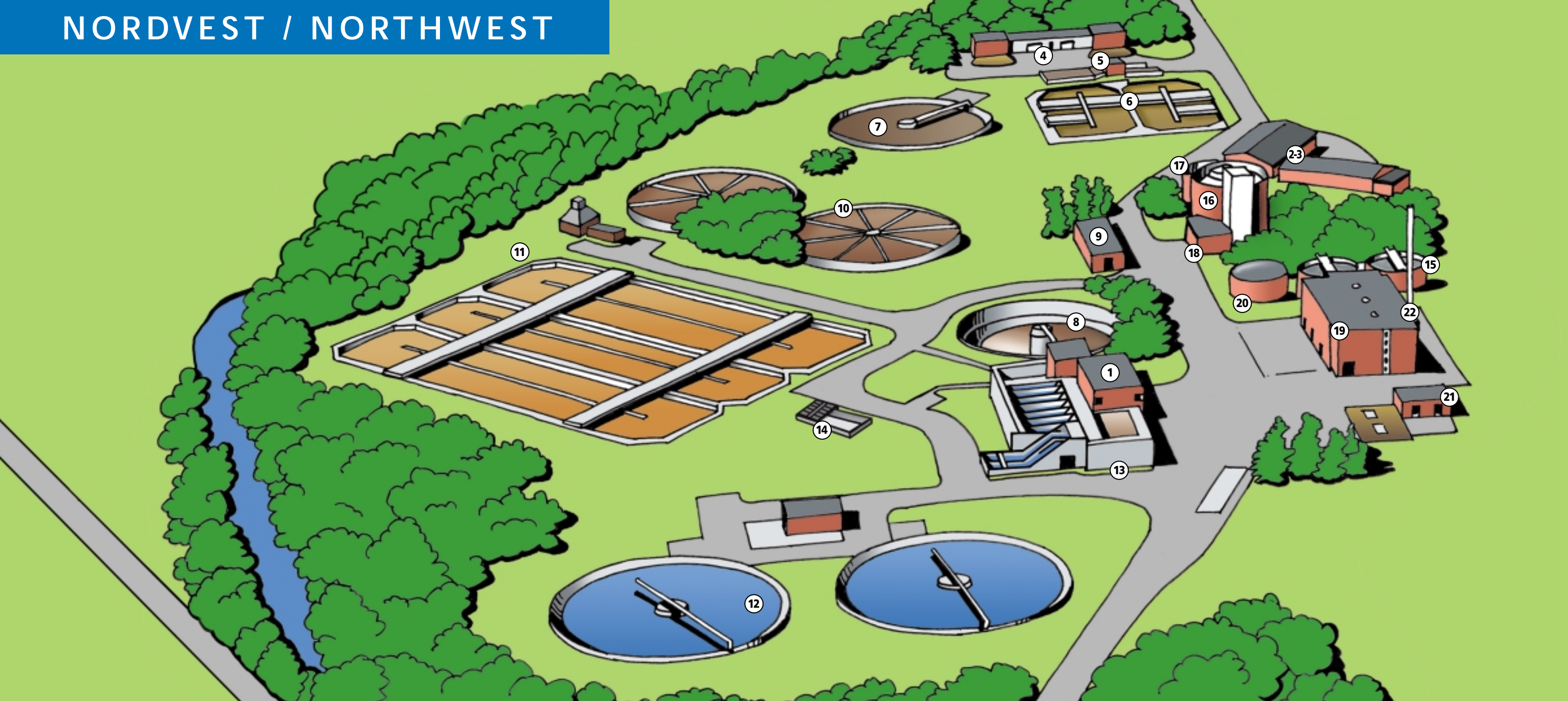
Riste og Sandfang Screens and grit chamber
